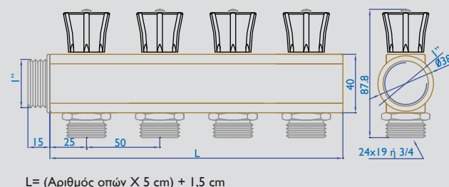
Συλλέκτης βολάν Α/Θ 1"
