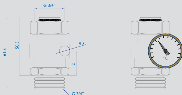
Μαστός επιστροφής
