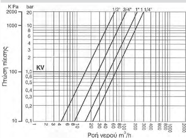
Διάγραμμα πτώσης πίεσης
