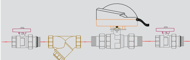
Υδραυλική Διάταξη
