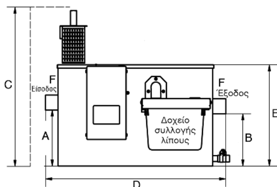
Πρόσοψη
