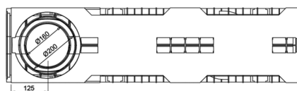
Κάτοψη: 200/160 + 200/100 + 200/40
