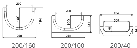
200/160 200/100 200/40
