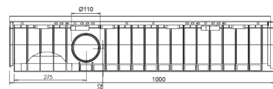
Πλάγια όψη 150/160
