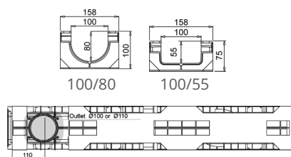
Κάτοψη: 100/80 + 100/55
