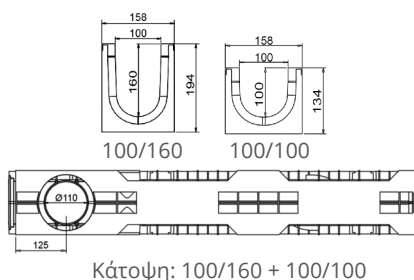
Κάτοψη: 100/160 + 100/100
