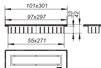
Cera Niveau brass matt
