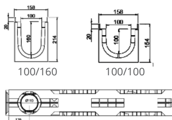
Κάτοψη: 100/160 + 100/100
