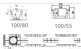
Κάτοψη: 100/80 + 100/55
