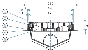
Πλάγια όψη
