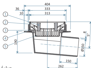
Πλάγια όψη
