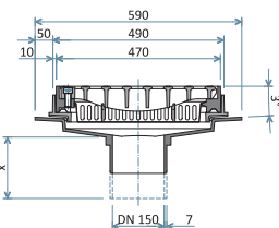
Πλάγια όψη
