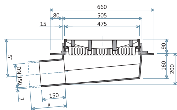
Πλάγια όψη
