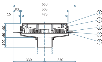
Πλάγια όψη
